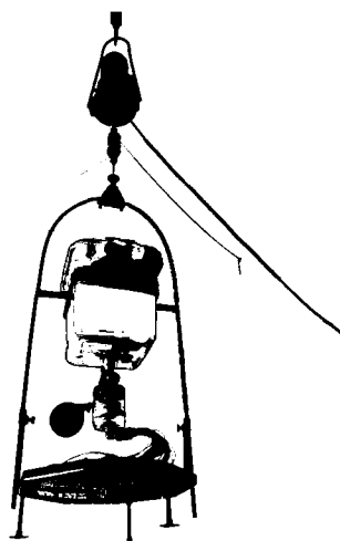
Рис. 2 – Портативная лабораторно-полевая дождевальная установка Fig. 2 – Portable laboratory-field rainfall simulator
